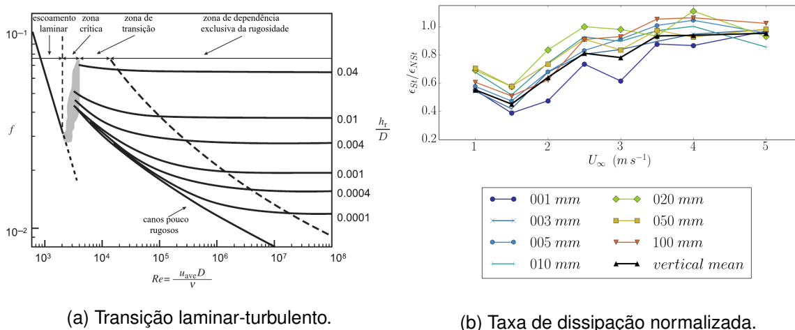
Figura 2 – Características do escoamento turbulento. A figura 2a mostra a transição de um escoamento laminar para turbulento. Adaptada de Wyngaard (2010, p. 5). A figura 2b apresenta o resultado encontrado neste estudo para a variação da taxa de dissipação com a velocidade do escoamento livre em um tunnel de vento.
